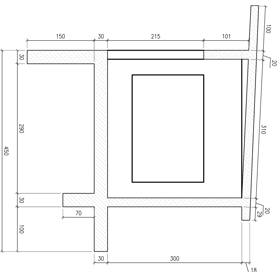
Przekrój G-G
