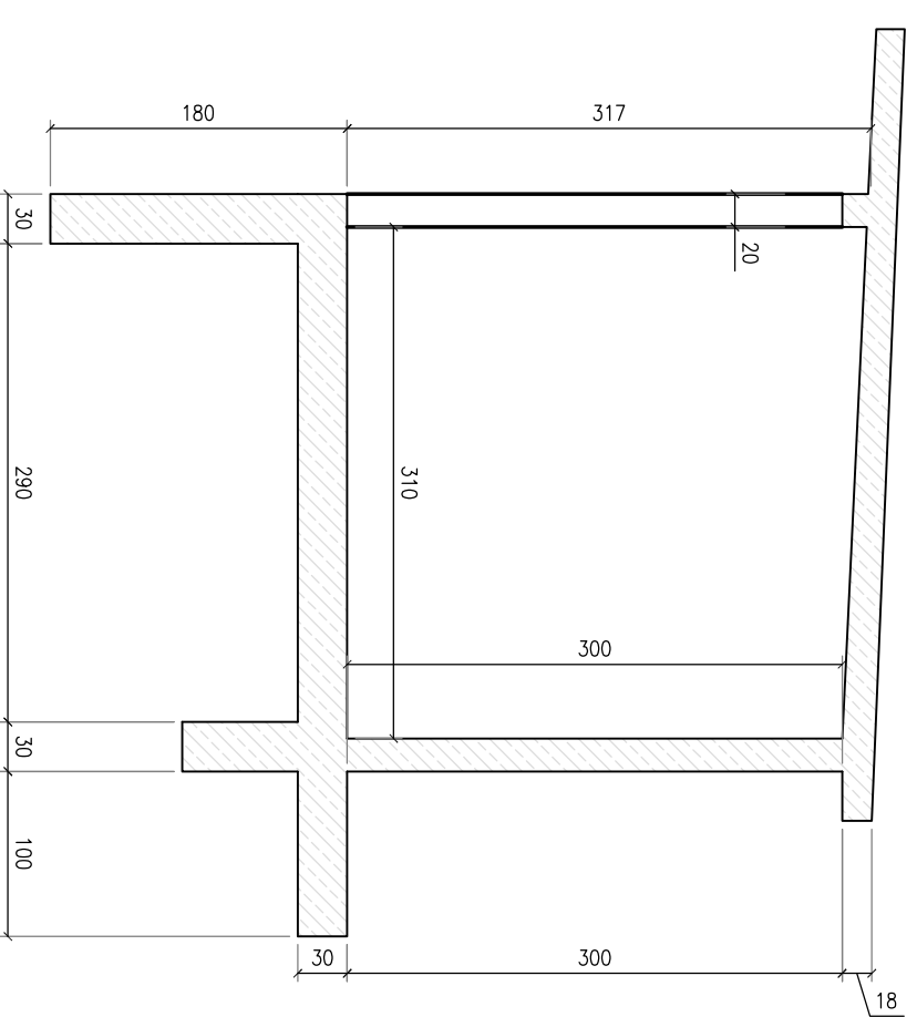
Przekrój H-H
