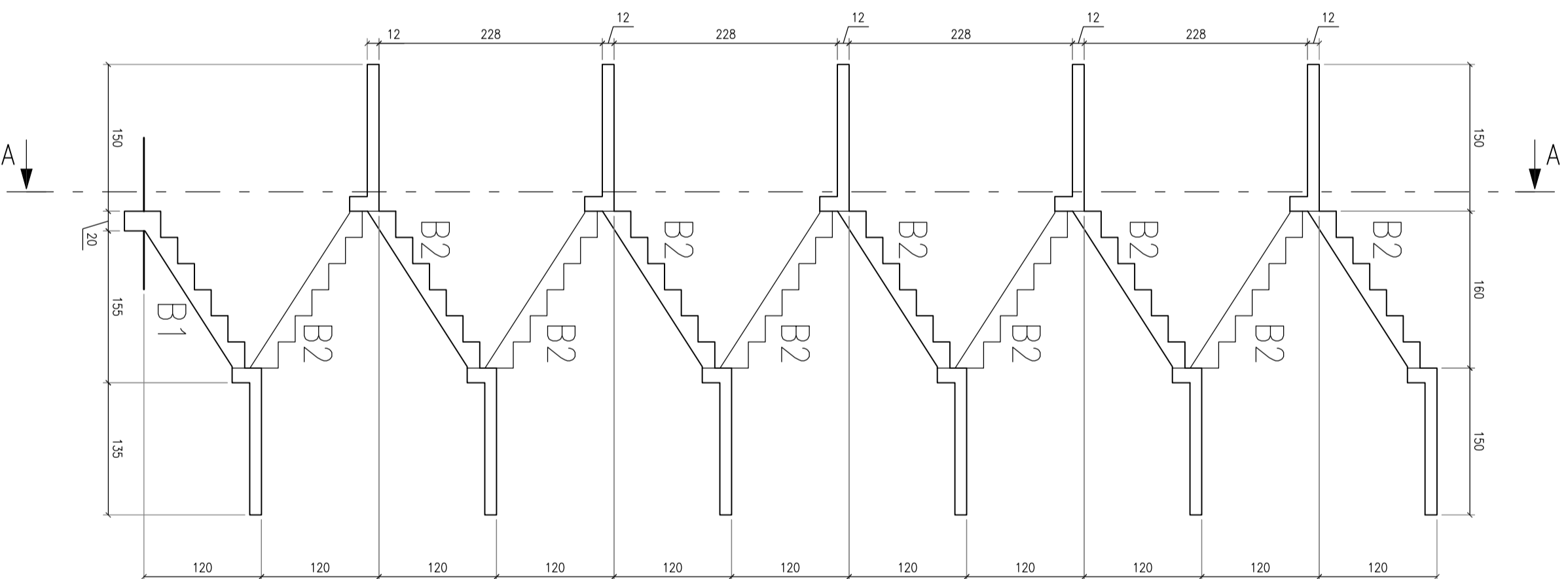
Przekrój B-B
