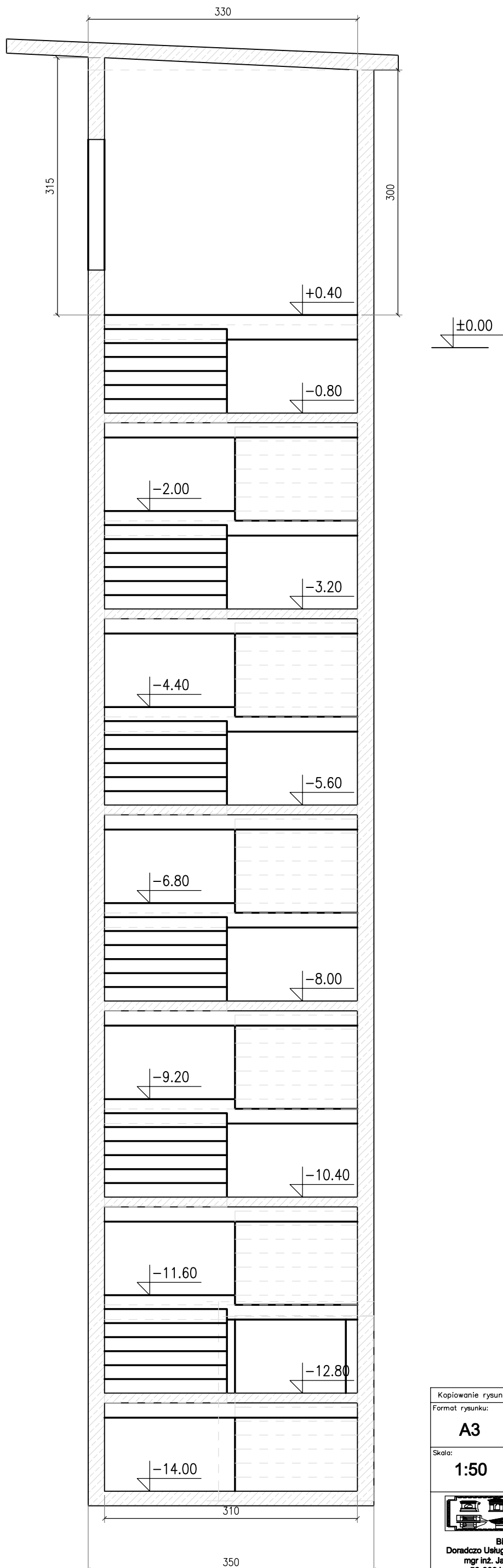
Przekrój D-D
